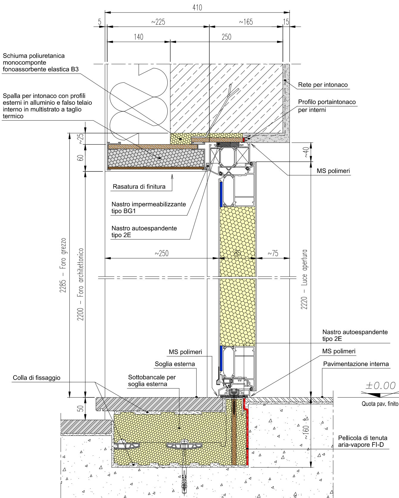
Sezione verticale tipo porte ingresso
