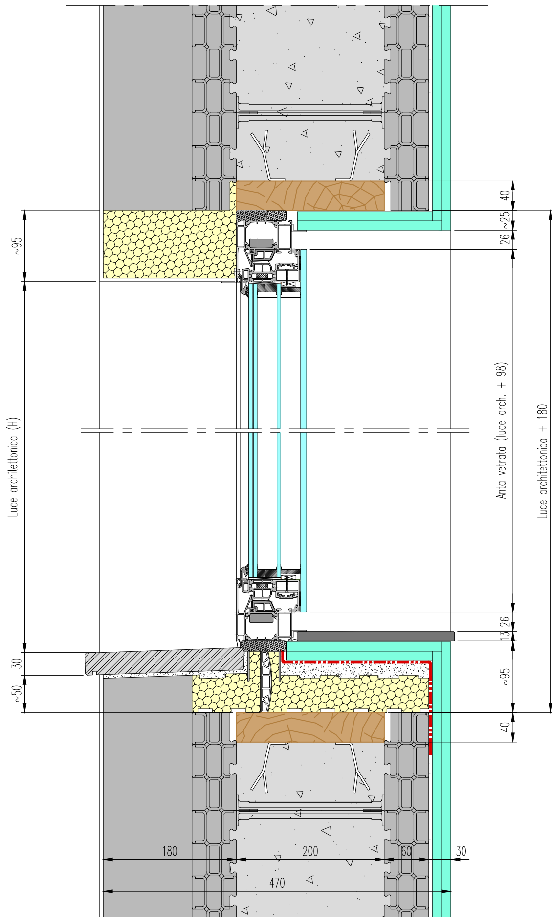
Sezione verticale tipo anta/ribalta
