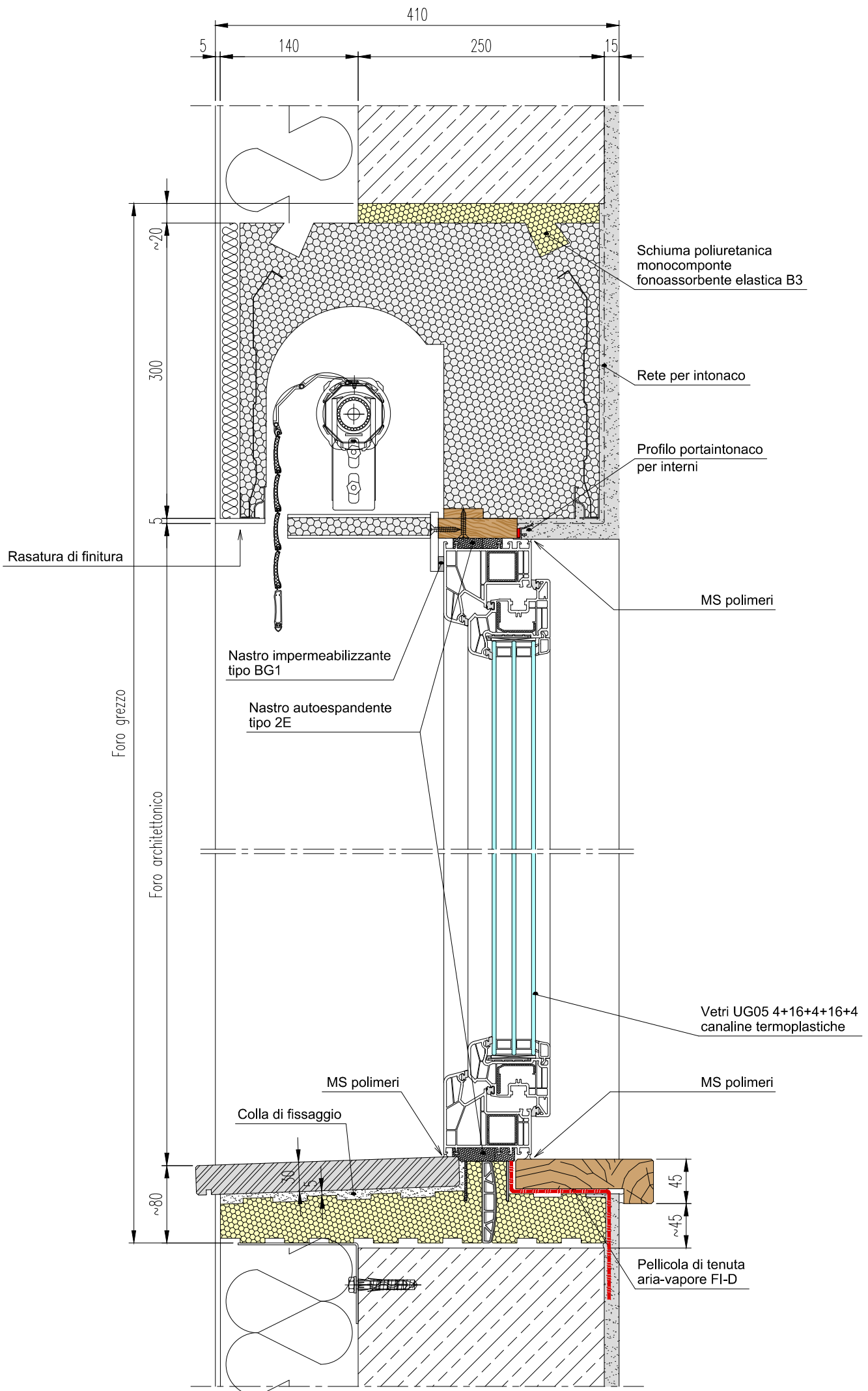
Sezione verticale tipo finestre
