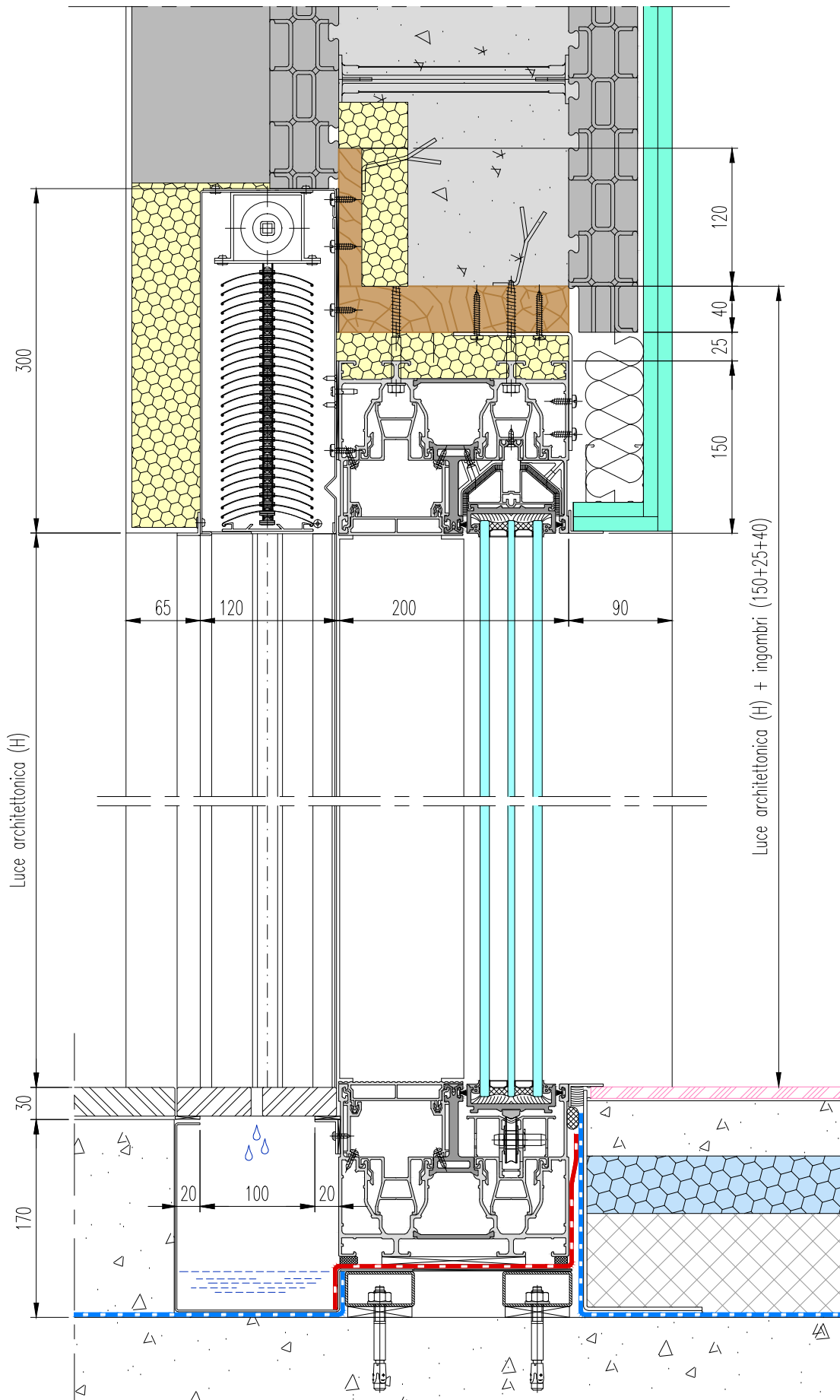
Sezione verticale tipo scorrevoli
